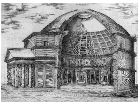
Slika 3: Prerez Panteona
